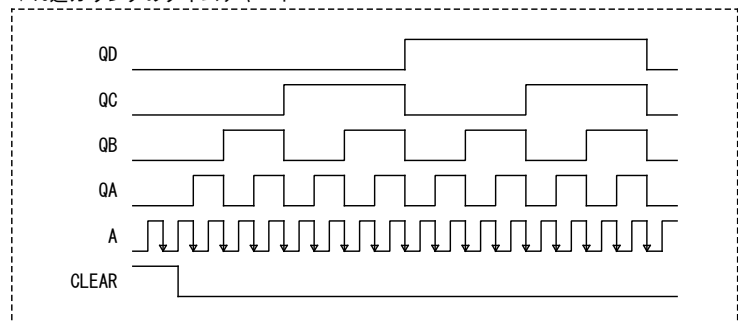
▼16進カウンタのタイムチャート
